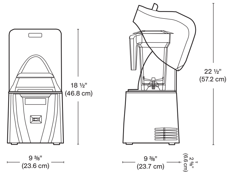
Figure 4. Connoisseur 825 Dimensions
